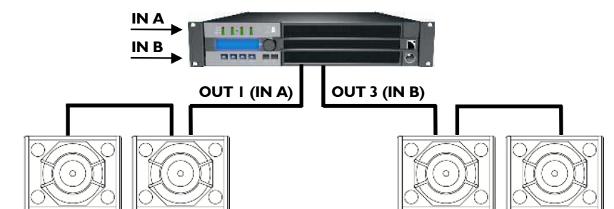
Figure 5 : Quatre enceintes I15XT HiQ connectées à un contrôleur LA8
