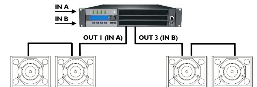
Figure 7 : Quatre enceintes I15XT HiQ raccordées à un contrôleur LA8
