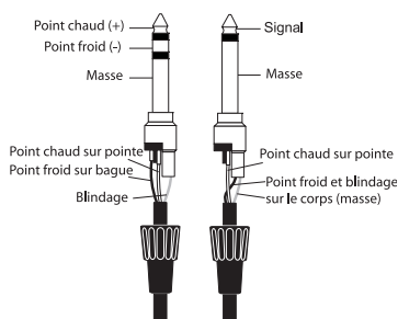
Jack stéréo symétrique
