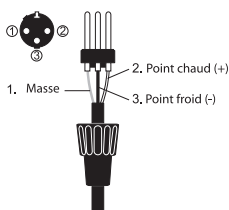
XLR micro symétrique
