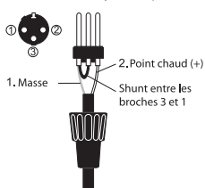
XLR micro asymétrique
