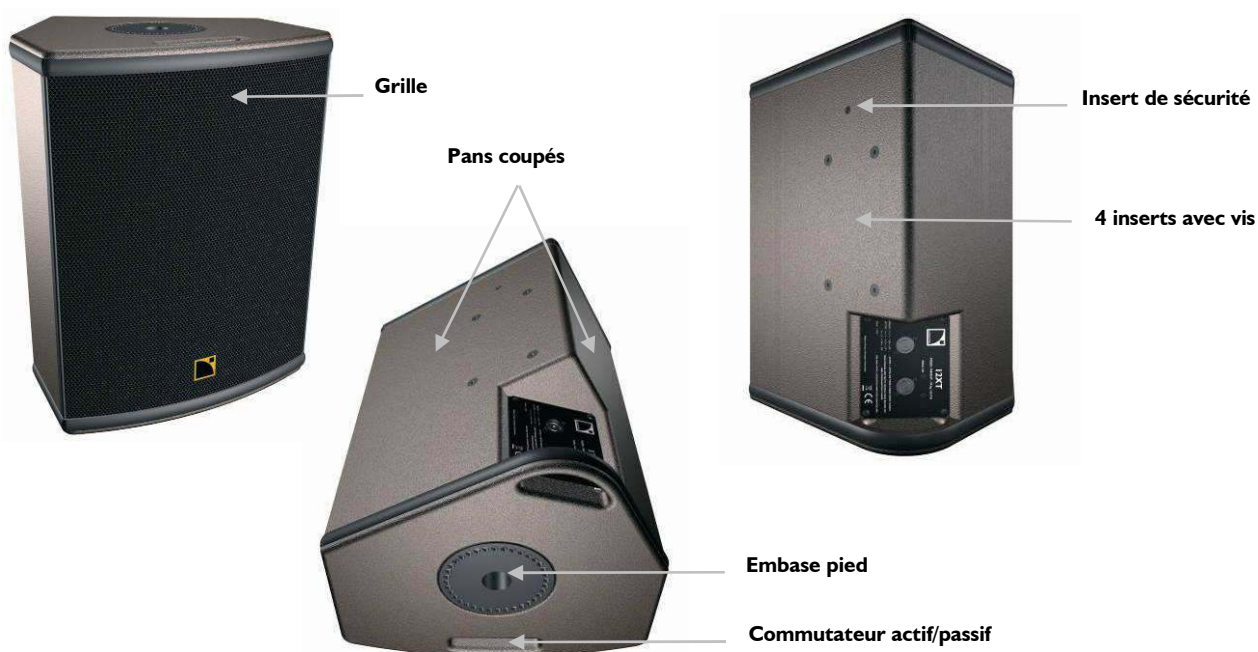
Figure 3 : L'enceinte 12XT
