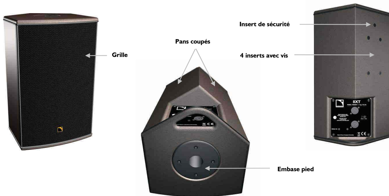
Figure 3 : L'enceinte 8XT
